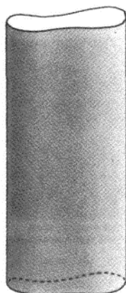
Weltfläche des geschlossenen String
