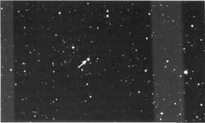
Abb. 20: Der durch den Pfeil gekennzeichnete Stern auf dem Foto ist Cygnus X-1, von dem man vermutet, er bestehe aus einem Schwarzen Loch und einem normalen Stern, die einander umkreisen.
