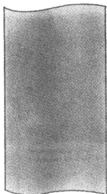
Weltfläche des offenen String
