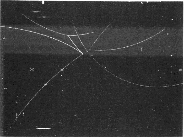
Abb. 18: Ein Proton und ein Antiproton kollidieren mit großer Energie und erzeugen einige fast freie Quarks. (Foto: CERN)
